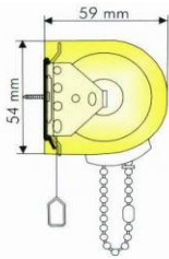
mit Trägerprofil
