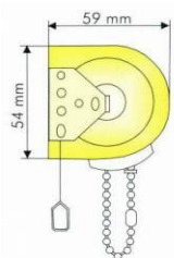
mit Montageträger
